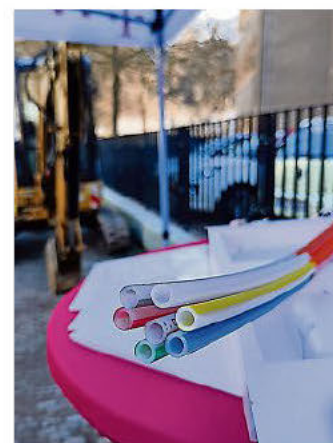
Innenleben Glasfaserkabel.
